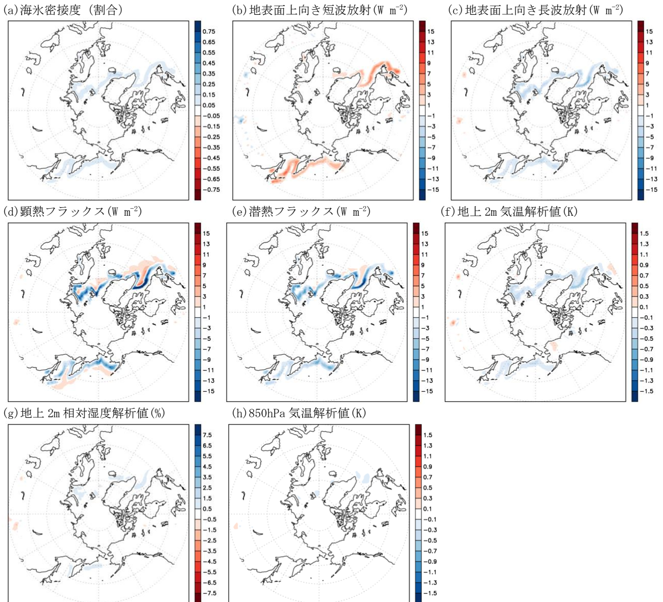
図2 北半球における海水氷接度の取扱い誤りによる影響 (2)
