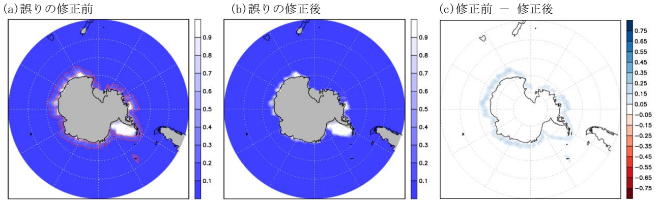
図3 南半球における海氷密度の取扱い誤りによる影響 (1)
