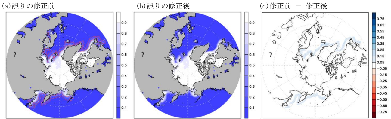
図1 北半球における海水氷接度の取扱い誤りによる影響 (1)
