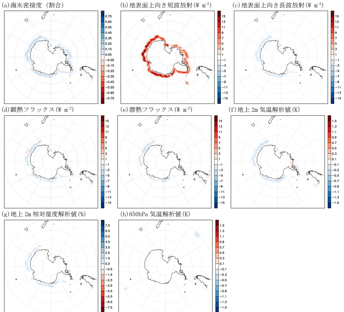
図4 南半球における海氷密度の取扱い誤りによる影響 (2)
